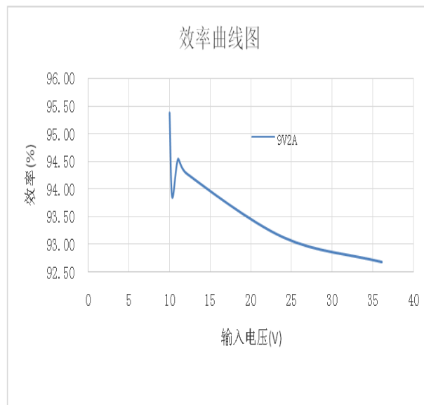
效率与输入电压特性曲线
