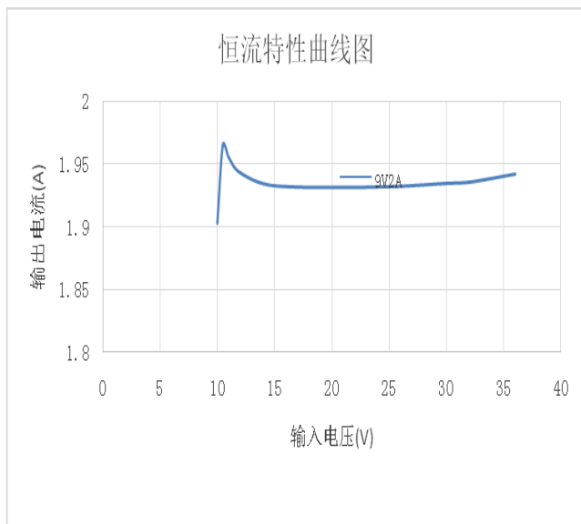
输出电流与输入电压特性曲线
