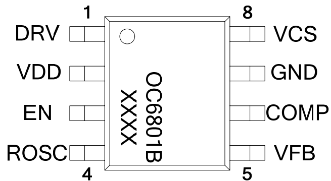
SOP8
