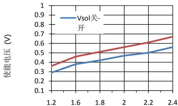
使能电压 vs. 输入电压
