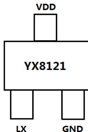
SOT23
