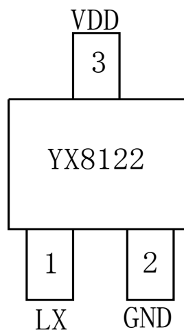
SOT23
