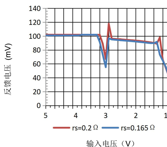
反馈电压 vs. 输入电压
