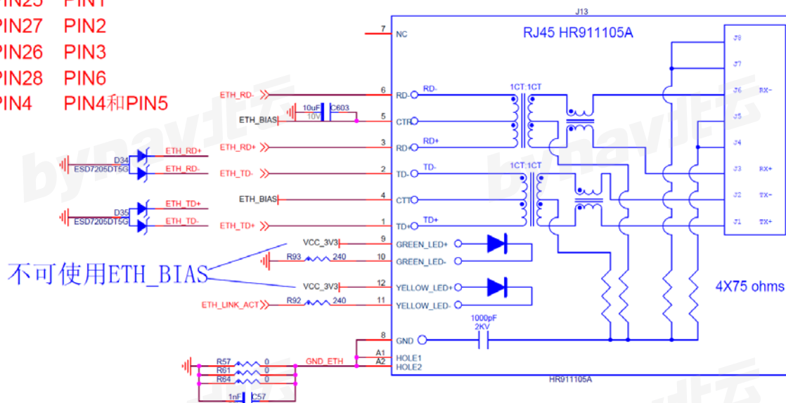
图 5 A1 板卡网口推荐电路
