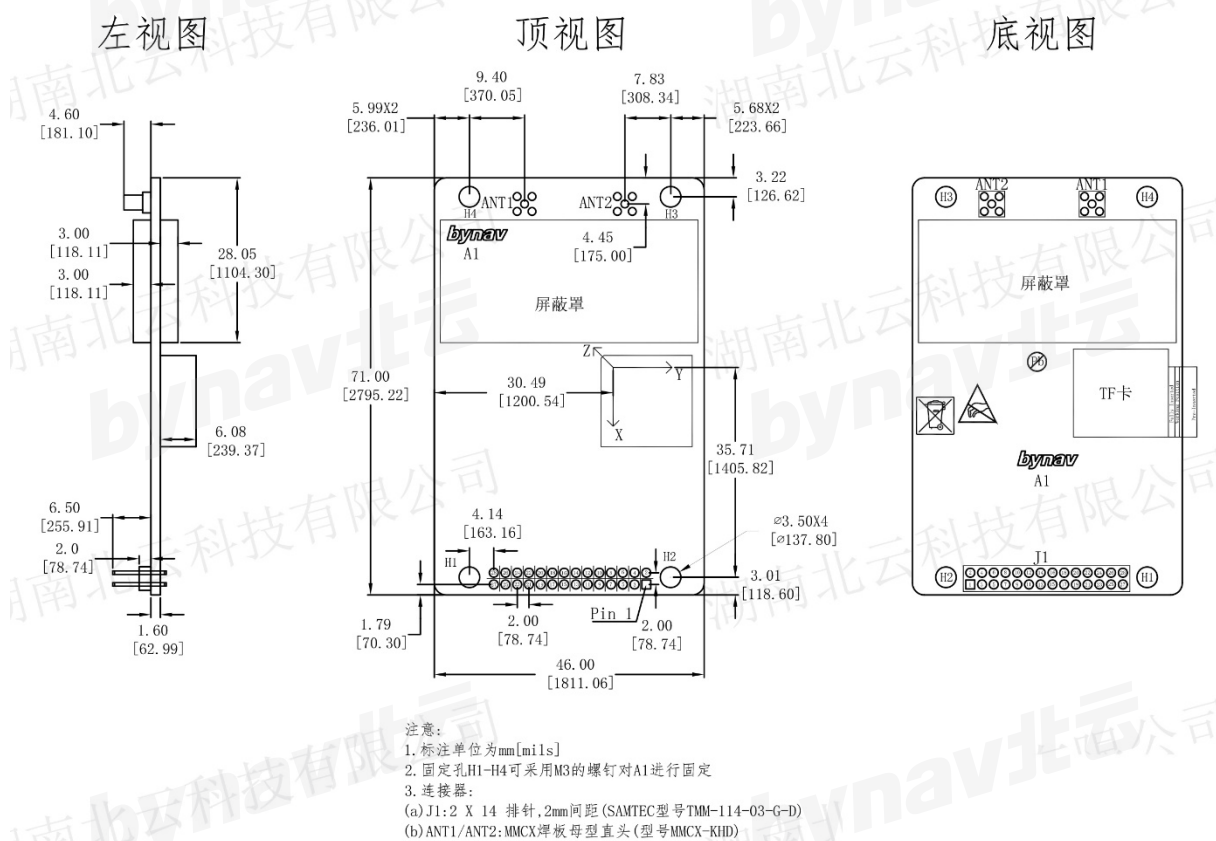
图 3 A1-3L/H 板卡孔位
