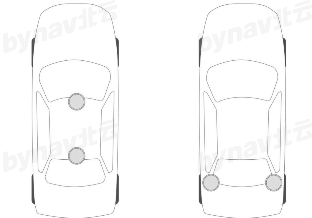
图 11 推荐的两种 GNSS 天线安装方式
