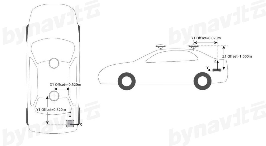
图 16 板卡到 GNSS 天线 1 的杆臂
