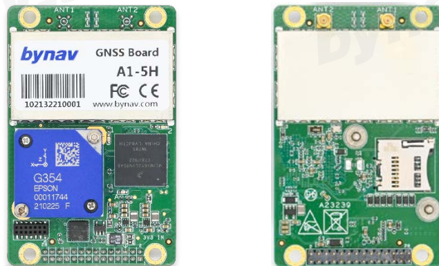
图 1 组合导航板卡 A1 外观图
