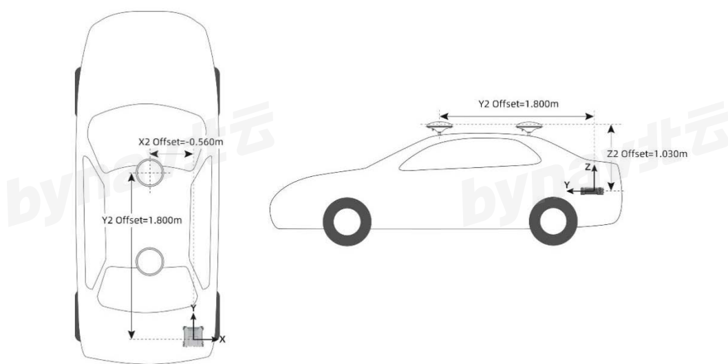
图 17 板卡到 GNSS 天线 2 的杆臂
